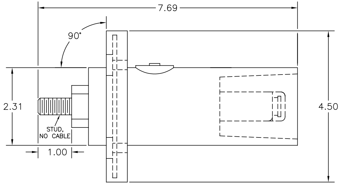
90° RECEPTACLE
