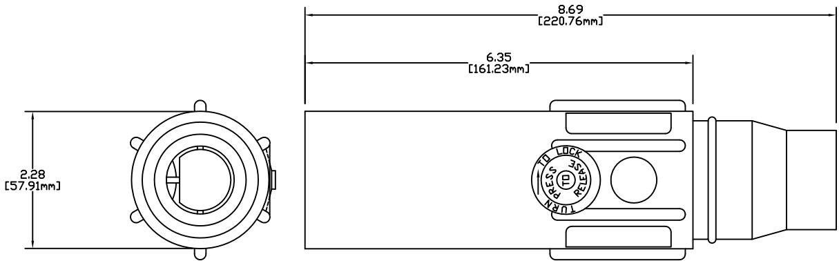
E1046, E1047, E1048, E1055, E1056, E1057 AND E1058 SERIES POSITIVE LATCHING LONG SHROUD POLARIZED MALE TAPERED NOSE MALE CONNECTOR 350 - 500 MCM CABLE VULCANIZED
