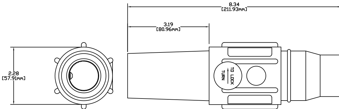
E1046, E1047, E1048, E1055, E1056, E1057 AND E1058 SERIES POSITIVE LATCHING LONG SHROUD POLARIZED FEMALE TAPERED NOSE FEMALE CONNECTOR 350 - 500 MCM CABLE VULCANIZED
